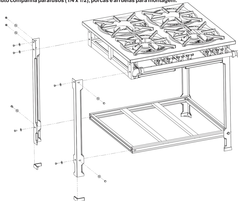
Modelo de tubo coletor de gás baixa pressão expandido:
