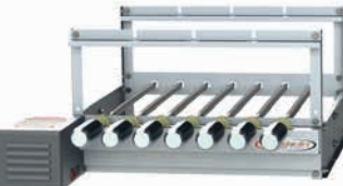
Itagrill Dupla Linear 7 Espetos * Espetos Espadas Altura: 28,5 cm Profundidade: 65,0 cm Frente: 48,5 cm Frente com Motor: 58,5 cm Código: 9326
