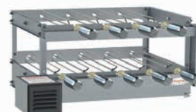
Itagrill Dupla 9 Espetos Altura: 31,0 cm Profundidade: 65,0 cm Frente: 60,0 cm Frente com Motor: 70,0 cm Código: 9213
