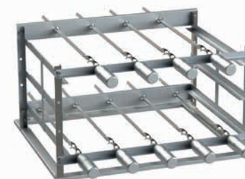
Suporte 9 Espetos Altura: 35,0 cm Profundidade: 52,0 cm Frente: 60,0 cm Código: 9161
