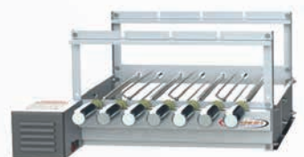
Itagrill Dupla Linear 7 Espetos * Espetos Mistos Altura: 28,5 cm Profundidade: 65,0 cm Frente: 48,5 cm Frente com Motor: 58,5 cm Código: 9323
