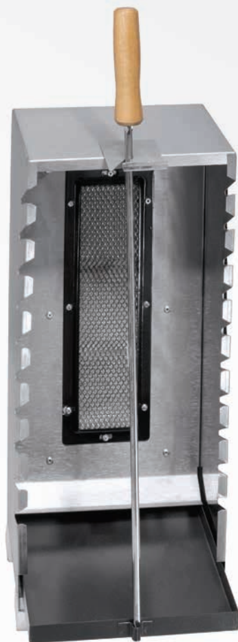
Itagrill Vertical Altura: 63,5 cm Profundidade: 35,5 cm Frente: 20,5 cm Código: 9159
