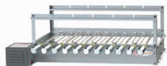
Itagrill Dupla Linear 11 Espetos * Espetos Mistos Altura: 28,5 cm Profundidade: 65,0 cm Frente: 71,5 cm Frente com Motor: 82,0 cm Código: 9321
