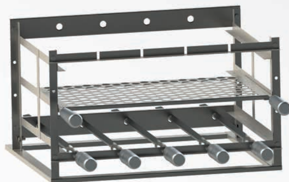
Suporte 5 Espetos Altura: 35,0 cm Profundidade: 52,0 cm Frente: 60,0 cm Código: 9200
