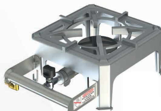
Fogão 1 Boca 1 Q. Simples Altura: 14,0 cm Profundidade: 36,0 cm Frente: 26,0 cm Código: 32140
