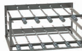
Suporte 11 Espetos Altura: 35,0 cm Profundidade: 52,0 cm Frente: 71,5 cm Código: 9160
