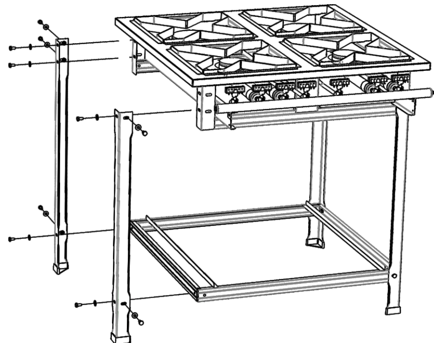
Modelo de tubo coletor de gás baixa pressão expandido:
