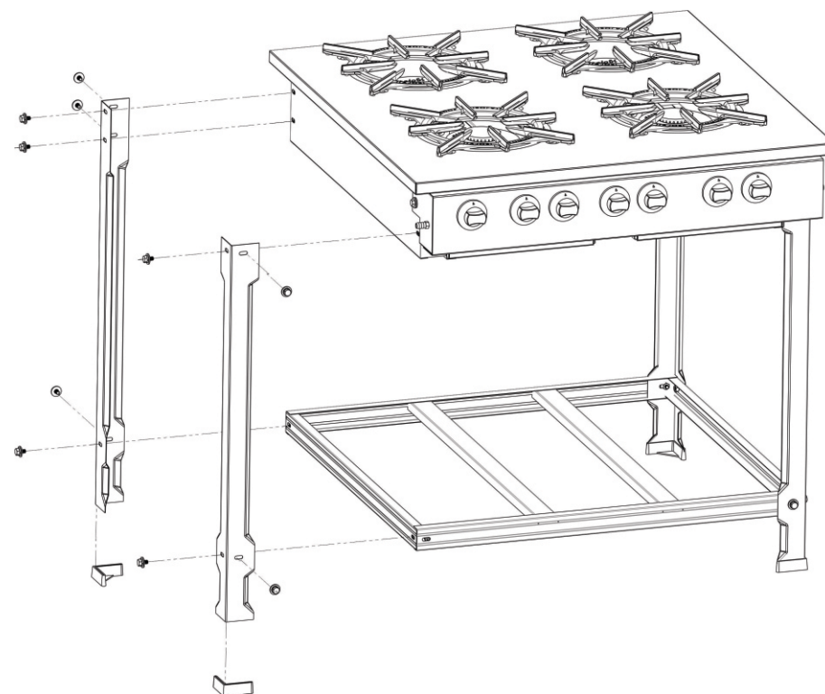
Modelo de tubo coletor de gás expandido:
